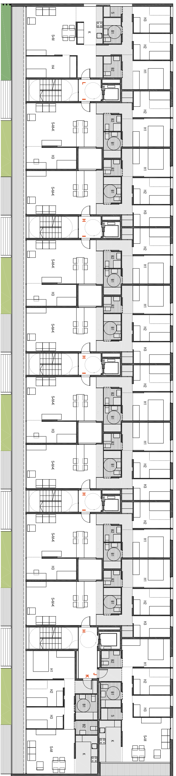
PLANTA TIPUS 1/ Bloc Carrer Malla Superfície Construída 995,30 m 2 11 Habitadges 1 Habitatge 4 dormitors 10 Habitadges 3 dormitors
