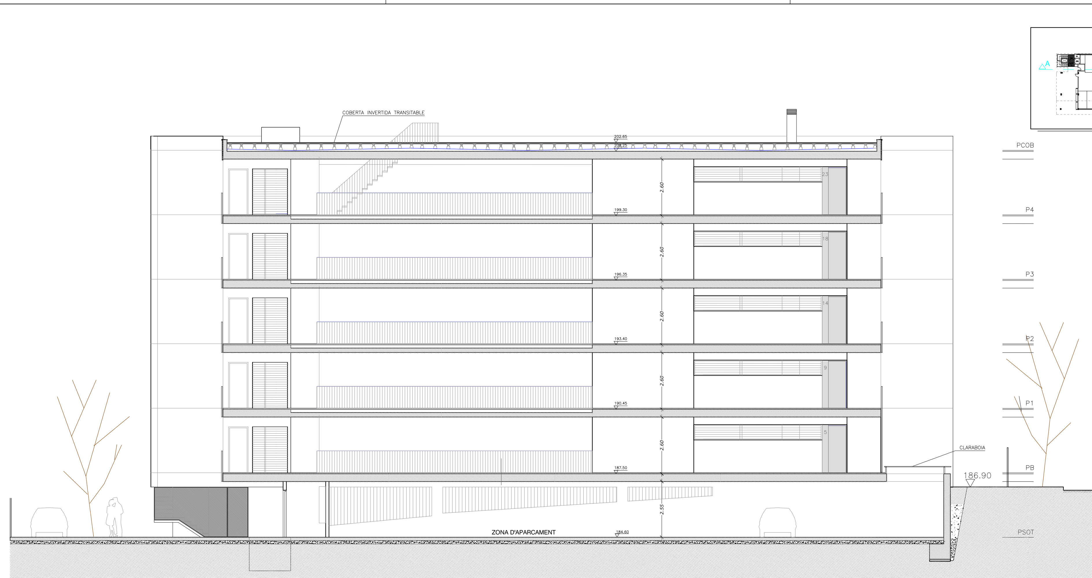
SECCIÓ A-A'
