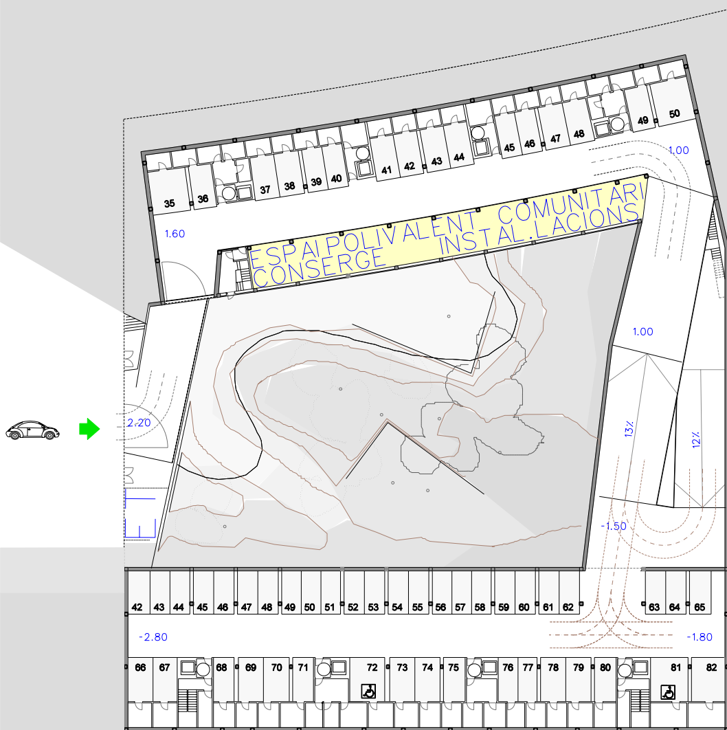
PLANTA SOTERRANI -2. APARCAMENT E. 1. 600
